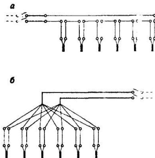
Рисунок 3. Схема электровзрывных цепей
