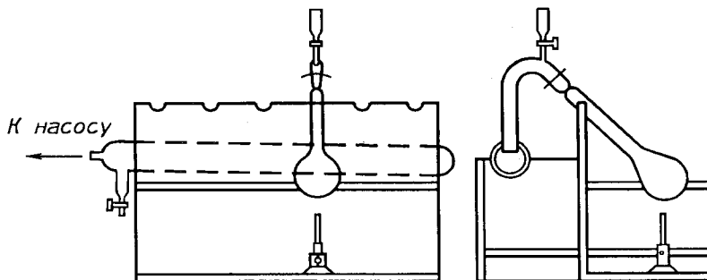
Рисунок 2 — Аппарат для мокрого окисления пробы
