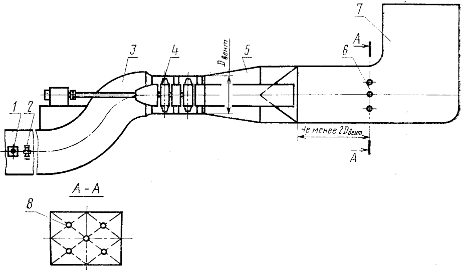
1—датчики давления вентилятора; 2—датчики подачи вентилятора; 3—канал вентилятора; 4—вентилятор; 5—диффузор; 6—измерительная поверхность; 7—выходная часть; 8—точки измерения
