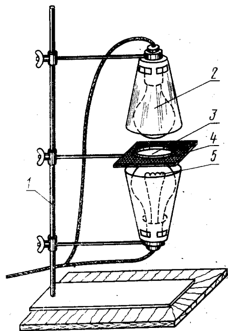
1—штатив; 2—рефлектор из жести; 3—алюминиевая чашка; 4—асбестовая сетка; 5—электрическая лампа.
