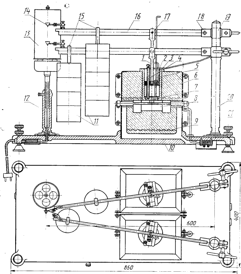
1—штемпель; 2—прижимная планка; 3—стакан; 4—трубка для терморары; 5—пластометр; 6—верхний кирпич; 7—дно стакана; 8—нагреватель; 9—нижний кирпич; 10—плата; 11—груз; 12—стойка барабана; 13—барабан с часовым механизмом; 14—перо; 15—подвеска груза; 16—рычаг; 17—шарнирный валок; 18—шарнирный валок; 19—муфта для крепления рычага; 20—стойка; 21—установочный винт
