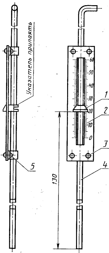
Пластометр
