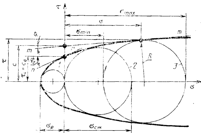
1 — круг одноосного растяжения; 2 — круг одноосного сжатия; 3 — круг объемного сжатия; pl — касательная к огибающей в точке ее пересечения с осью \tau ; mt — касательная к огибающей в любой точке на ней
