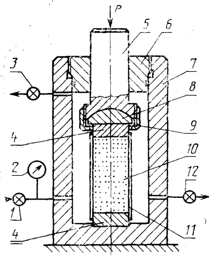
1 — впускной вентиль; 2 — манометр; 3 — вентиль выпуска воздуха; 4 — стальные плиты; 5 — шток; 6 — крышка; 7 — корпус; 8 — сферическая гайка; 9 — накидная гайка; 10 — образец; 11 — изоляция; 12 — выпускной вентиль
