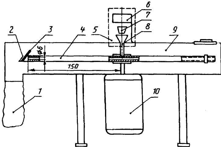
Рисунок 1 — Центробежный абразивметр
