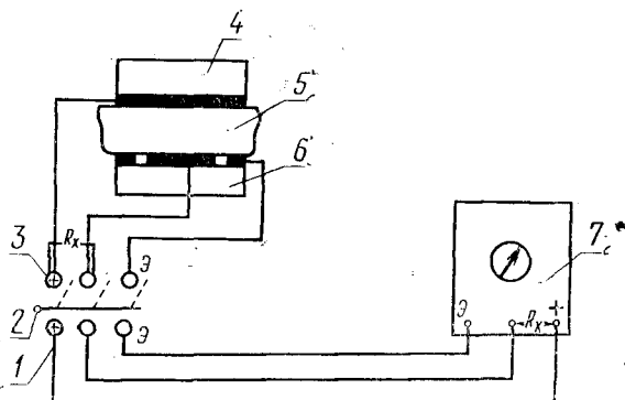
1—переносные контакты измерительного прибора; 2—ключ; 3—контакты измерительного устройства; 4—потенциальный электрод; 5—образец; 6—измерительный электрод; 7—измерительный прибор.
