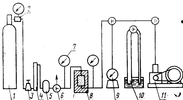
Принципиальная схема установки для определения газопроницаемости
