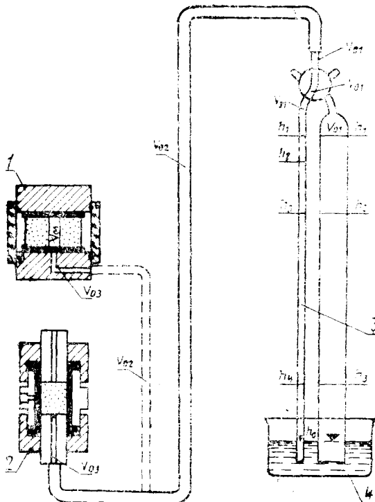
1—кернодержатель радиальный; 2—кернодержатель линейный; 3—двухрубный пьезометр; 4—сосуд для жидкости
