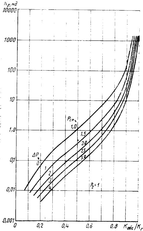
Номограмма для вычисления поправки к газопроницаемости за счет скольжения газа
