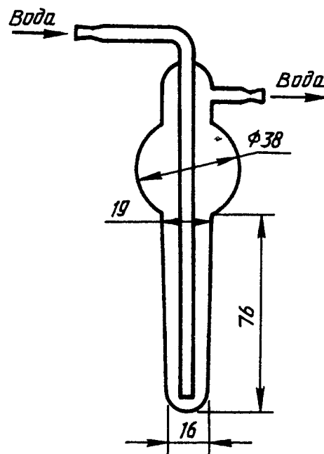
Рисунок 2 — Пальчиковый холодильник
