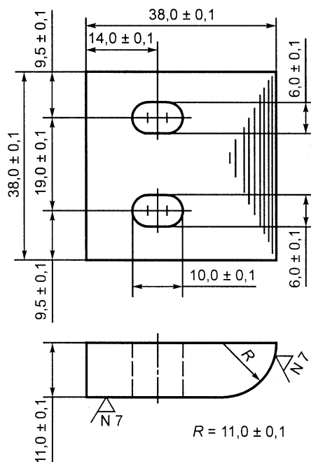
Рисунок 2 — Стальной нож
