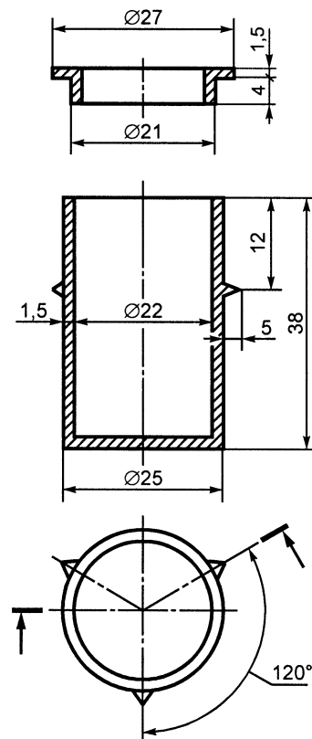
Рисунок 2 — Кварцевый тигель с крышкой
