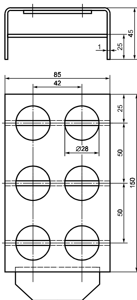
Рисунок 4 — Подставка для тиглей из листовой стали
