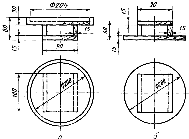
Рисунок 4 — Матрица для отжатаия влаги
