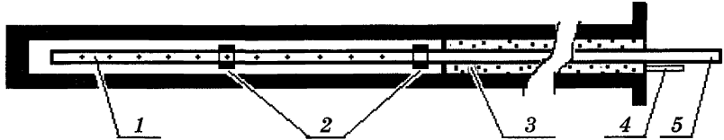
Рис. 9.1. Схема герметизатора:
