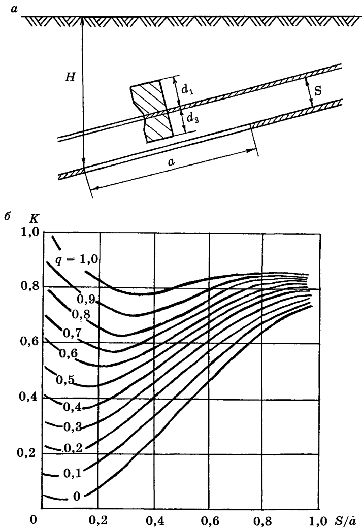
Рис. 5.11. Номограмма для определения влияния под- или надработки на параметры зон ПГД:
