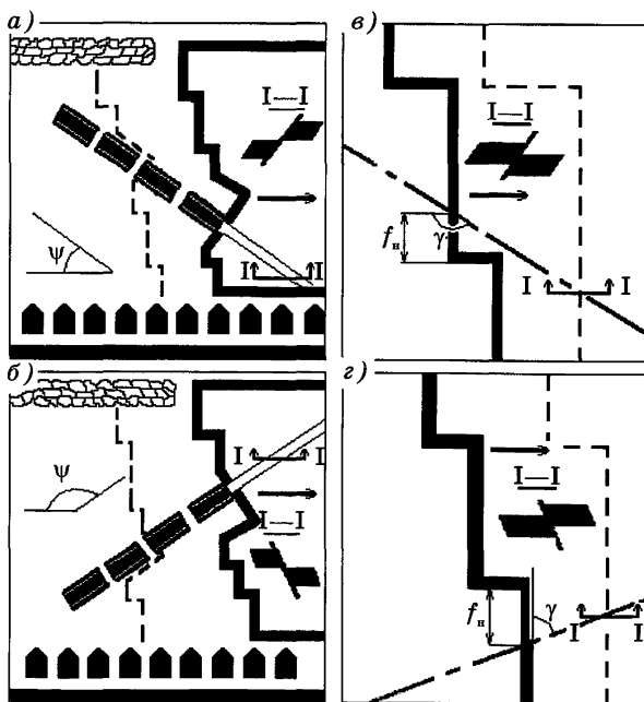
Рис. 14. Схемы перехода разрывных нарушений на круглых пластах:
