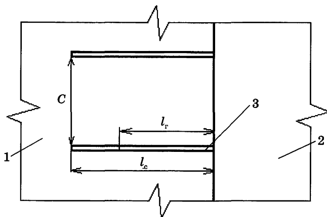
Рис. 9.5. Схема расположения шпуров для гидростатического сжатия пласта: 1 — участок пласта; 2 — выработанное пространство; 3 — нагнетательные скважины
