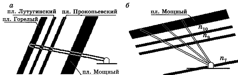
Рис. 9.2. Принципиальные схемы регионального увлажнения угольных пластов: а — АО «Проктопьевскуголь»; б — АО «Воркугауголь»
