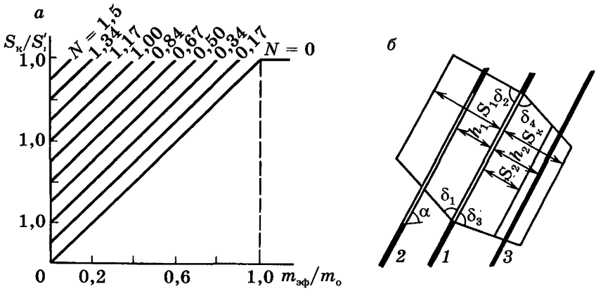
Рис. 5.6. Номограмма (а) и схема (б) к построению защищенной зоны при повторной надработке (подработке):
